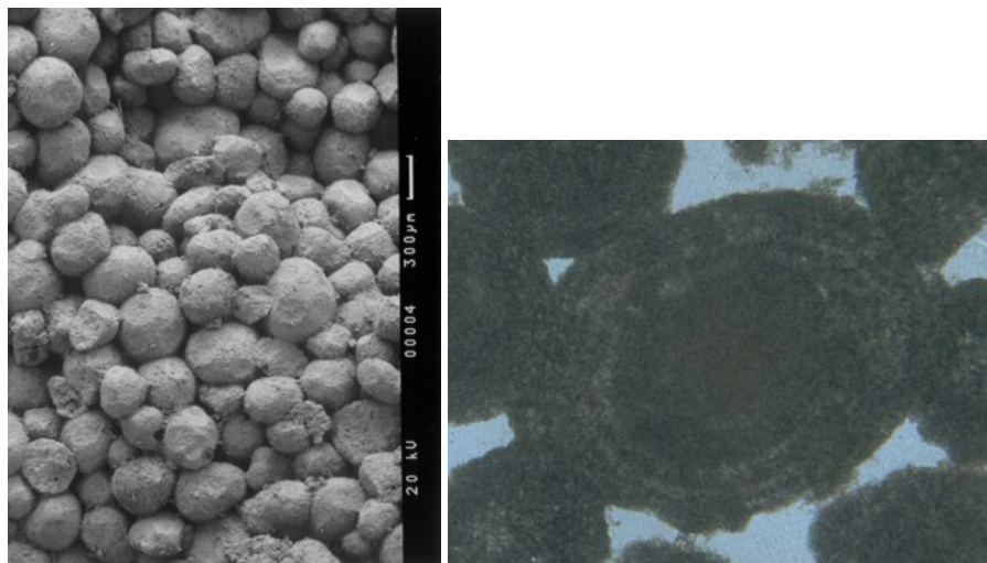
Slike 5.-6. Oolitična struktura tenelije (SEM snimka - LGA Nürnberg), lijevo; Tenelija: koncentrična struktura ooida (desno)
