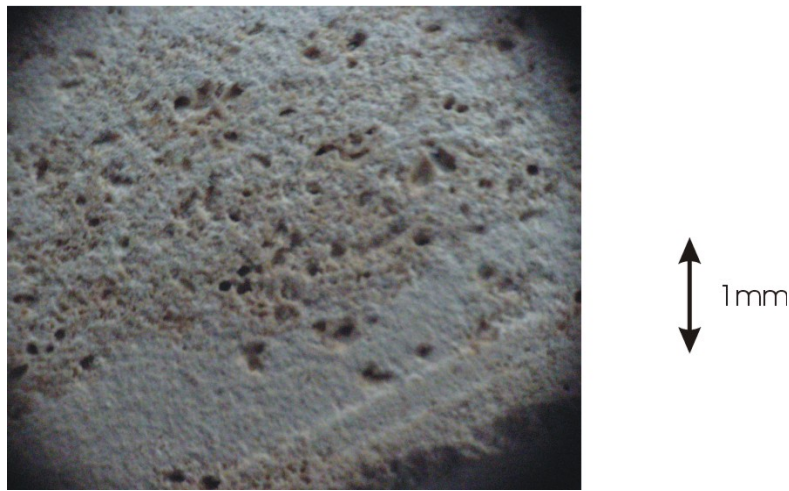
Slika 8. Sitnozrnata struktura miljevina (SEM snimka – LGA Nürnberg)
